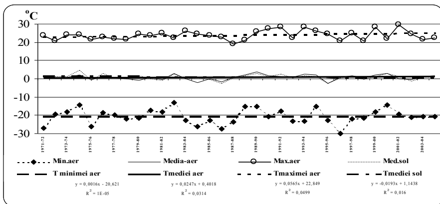
Fig. 2. Evoluția parametrilor termici principali în timpul semestrelor reci ale anului la Suceava (1971 – 2005).
